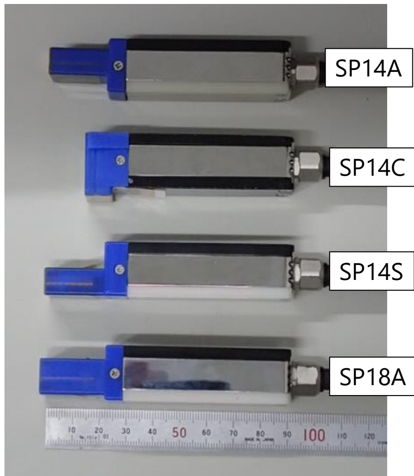
図1.センサープローブ外観
